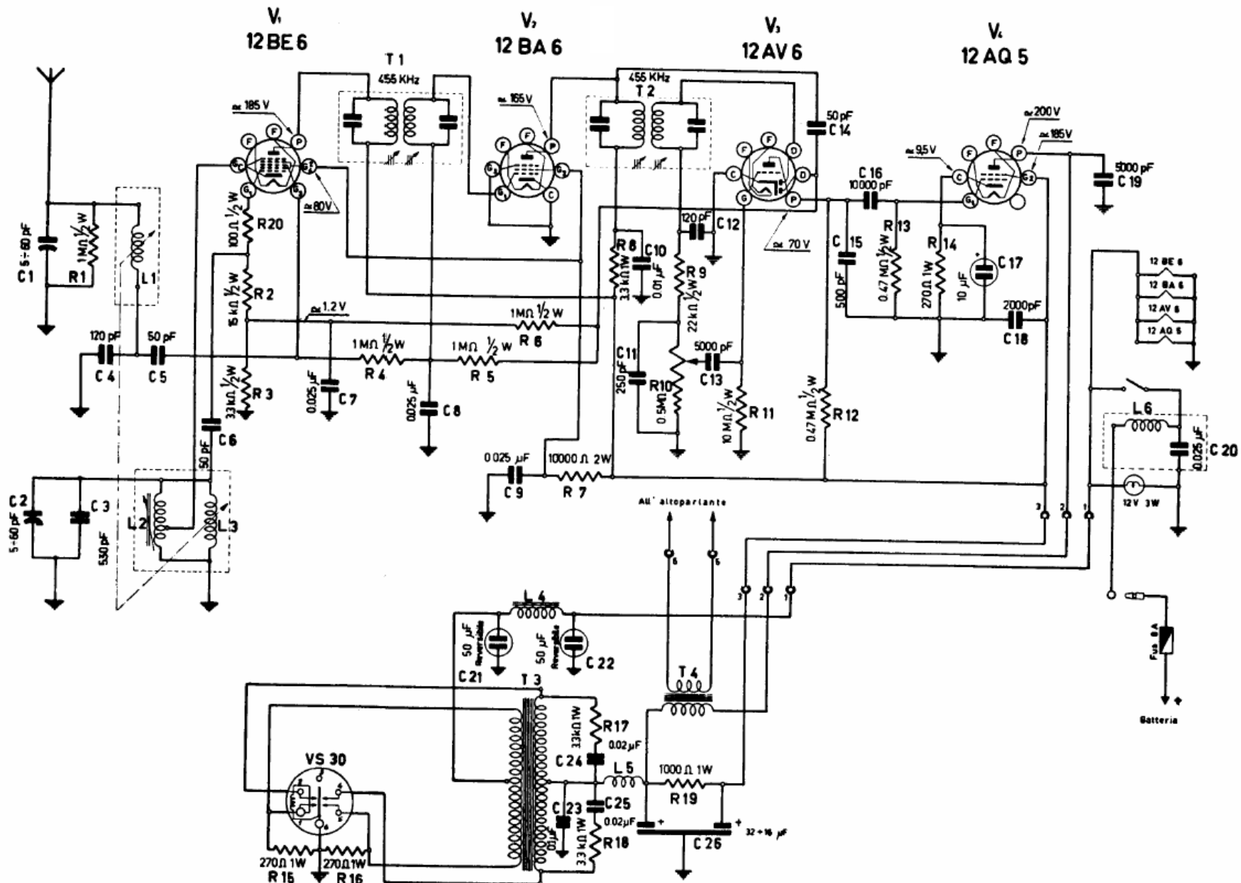
SCHEMA ELETTRICO DEI RADIORICEVITORI RA 90 E RA 91
